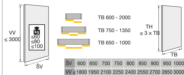
Materijal vrata
