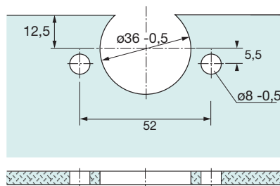
Šablona stak. vrata za čašicu T 22
