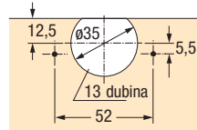
Šablona TH 32
