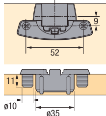
Šablona TX 33
