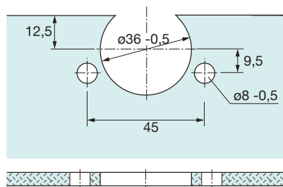
Šablona stak.vrata za čašicu TB 22
