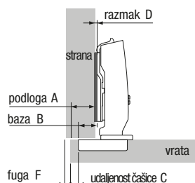
Šablona bušenja Sensys tanka vrata ŠV52
