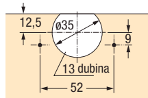
Šablona TX 32
