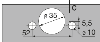
Šablona bušenja Sensys 165° 8657 TH 52
