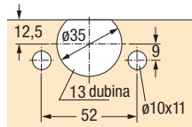
Šablona TX 33
