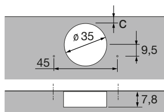
Šablona bušenja Sensys tanka vrata ŠV52
