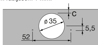
Šablona bušenja Sensys tanka vrata VV 52
