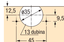
Šablona TB 32
