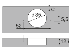
Šablona Sensys 12,9 mm TH 52
