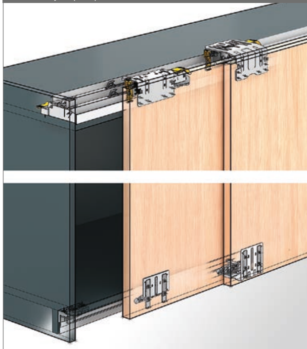
Konstrukcijski princip
