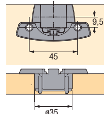
Šablona TB 32
