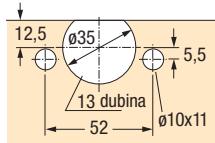
Šablona TH 33
