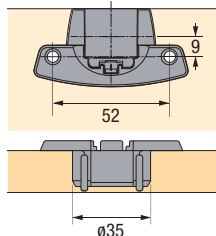
Šablona TX 32
