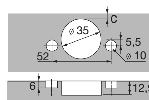
Šablona Sensys 12,9 mm THS 55
