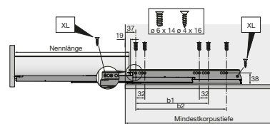
Montaža AvanTech You ladica
