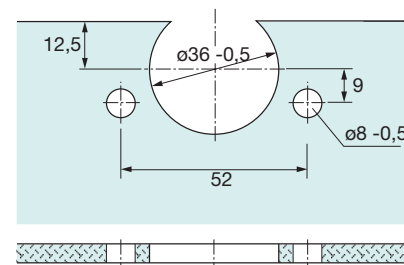
Šablona stak.vrata za čašicu T22/9
