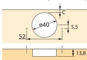
Mjere bušenja T22/40
