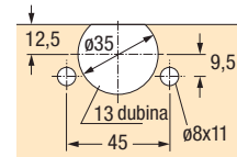
Šablona TB 33
