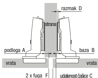
Šablona bušenja Sensys tanka vrata VV 58
