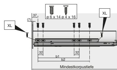
Montaža AvanTech You unutarnjih ladica
