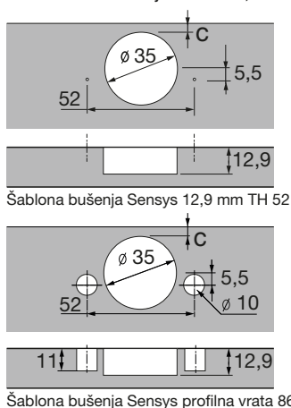
Šablona bušenja Sensys profilna vrata 8631i Flash
