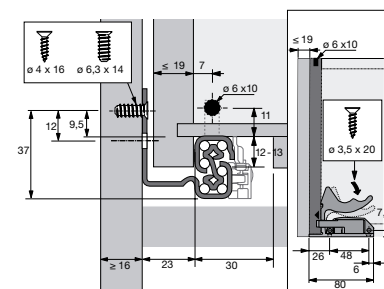
Dno s utorom
