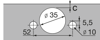
Šablona bušenja Sensys tanka vrata VV 58
