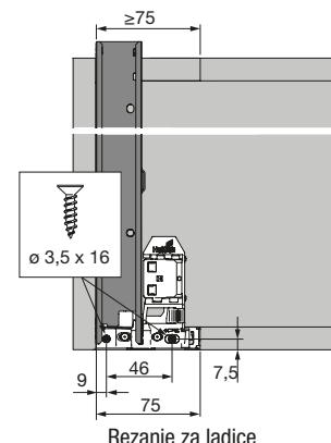
Rezanje za ladice
