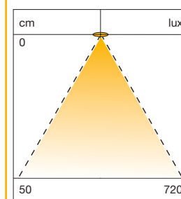
Dijagram raspodjele svjetlosti
