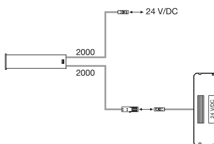
Priključak 24 V/DC
