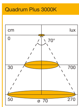
Dijagram raspodjele svjetla
