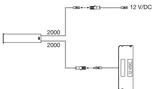
Priključak 12 V/DC
