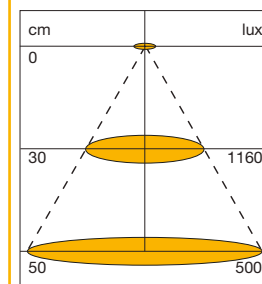
Dijagram raspodjele svjetlost
