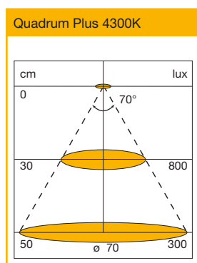
Dijagram raspodjele svjetla
