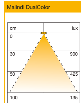
Dijagram raspodjele svjetla
