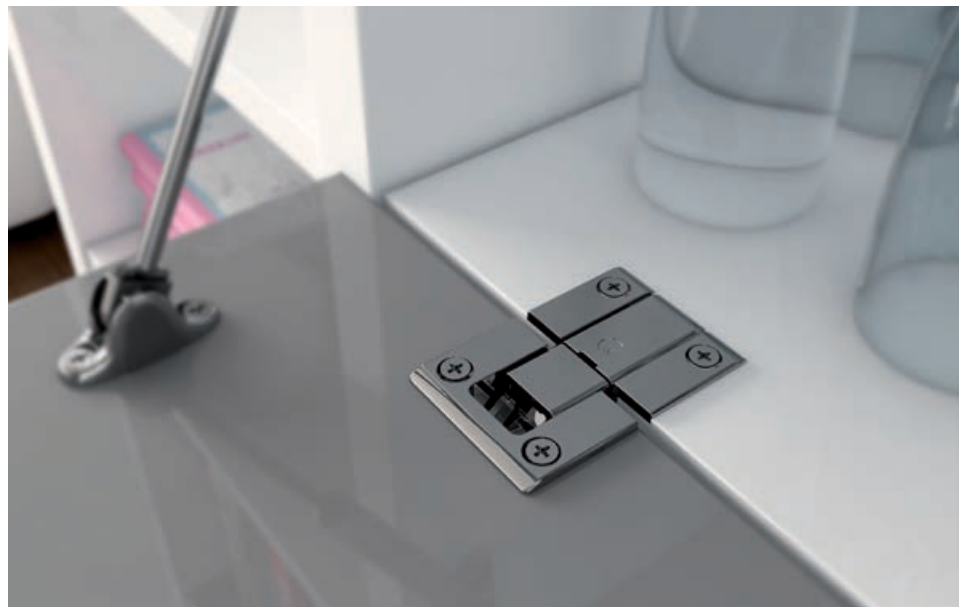
Varijanta: debljina fronte 19 mm; debljina korpusa 16 mm
