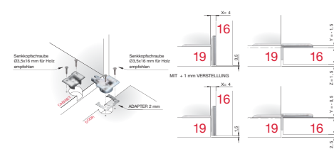
Varijanta: debljina fronte 16 mm; debljina korpusa 19 mm
