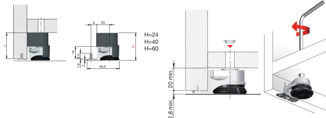
Montaža vijcima
