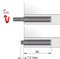
Verstellung
