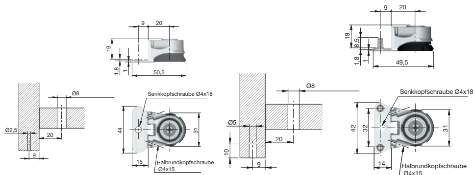
Montaža vijcima
