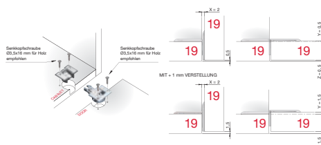
Varijanta: debljina fronte 19 mm; debljina korpusa 19 mm
