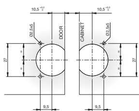
Varijanta: debljina fronte 19 mm; debljina korpusa 16 mm
