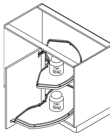
Ausführung: rechts
