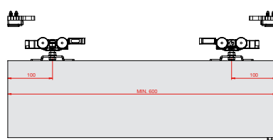
Montaža kotačića Classic Basic Standard
