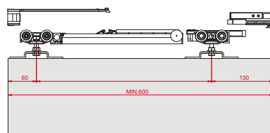
Pozicija montaže kotačića Classic Fluid / Basic Komfort
