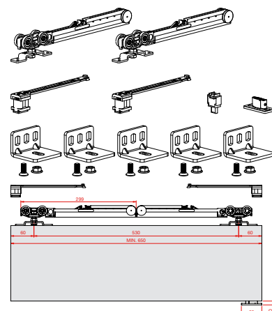
Pozicija montaže kotačića Classic Fluid 50
