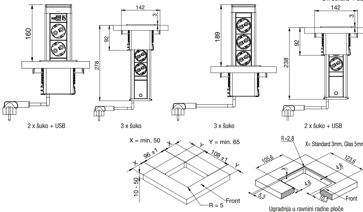
2 x Schuko + USB punjač, poklopac crni
