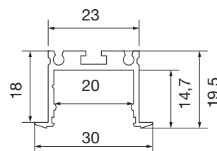
Profil s pokrovom i završnim kapicama
