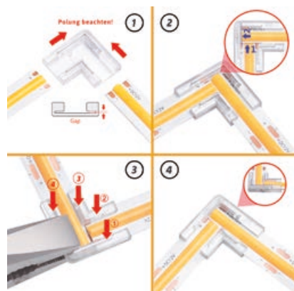
Obrada kutnog veznika
