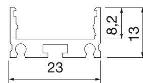
Profil s pokrovom i završnim kapicama
