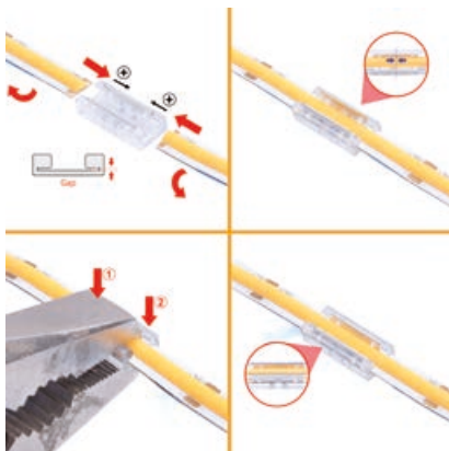
Obrada izravnog veznika
