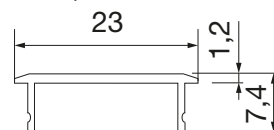
Profilni pokrov SX09
