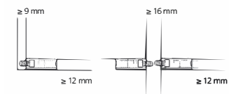
Cabineo vijak 8
