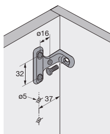
❸ Upuštena leđa ormara, pričvršćivanje s Panhead ø 4 x 12 mm
