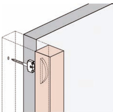
Primjena završna lajsna
