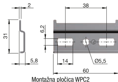
Montažna pločica WPC2
