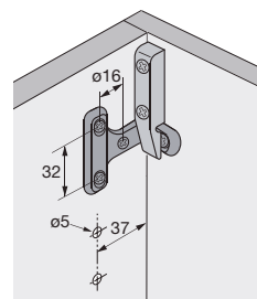
❺ Tupo naliježuća leđa ormara, pričvršćivanje s MultiClip
