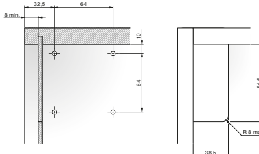
Mjere kod primjene bez pokrova
