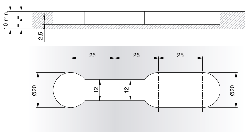
Alternativni plan bušenja
