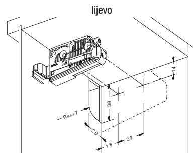
pričvršćivanje vijcima
