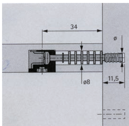
ugradbena mjera sredina ekscentra 34 mm
