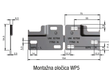
Montažna pločica WP5
