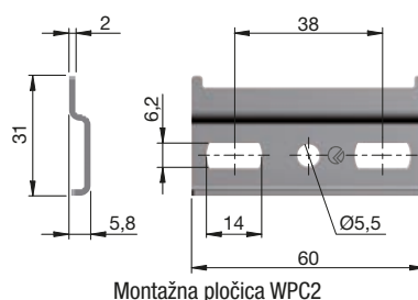
Montažna pločica WPC2
