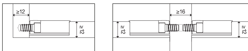
Primjena Cabineo 8 M6
