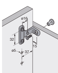
❷ Tupo naliježući Leđa ormara (min. 16 mm), Pričvršćivanje lečastim vijkom M6 x 12 (DIN 7985) s kapicom s navojem M6
