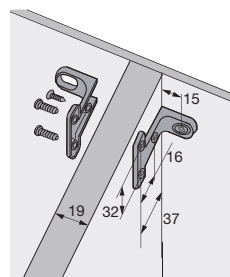
❹ Pričvršć. srednjeg zida s Panhead ø 4 x 12 mm
