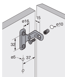
❶ Tupo naliježući Leđa ormara (min. 16 mm) Pričvršćivanje lečastim vijkom M6 x 12 (DIN 7985) i čahurom
