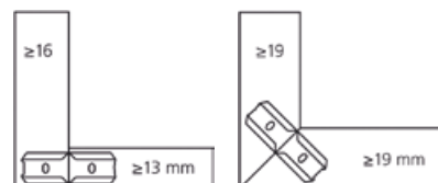
Različiti kutni spojevi od 30°-180°
