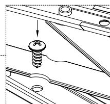
Limitatore Limiter
